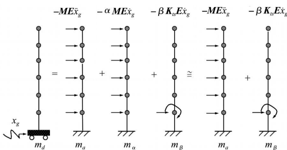
图 1 位移输入模型等效分解示意图 Fig. 1 Equivalent sketch of displacement input model
