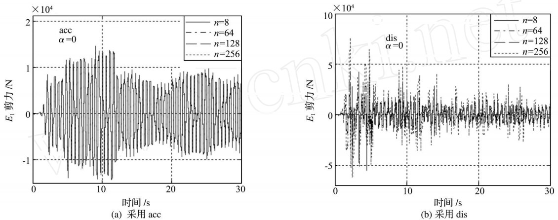
图 7 n 不同取值时 E_1 剪力比较 ( \alpha = 0 )
