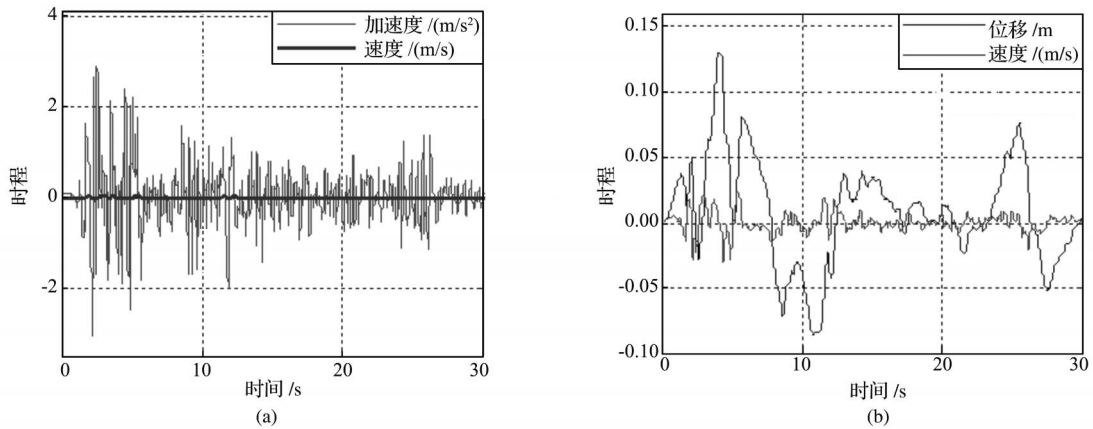
图 3 El Centro 波时程曲线(1940) Fig. 3 Time history curves of El Centro (1940)
